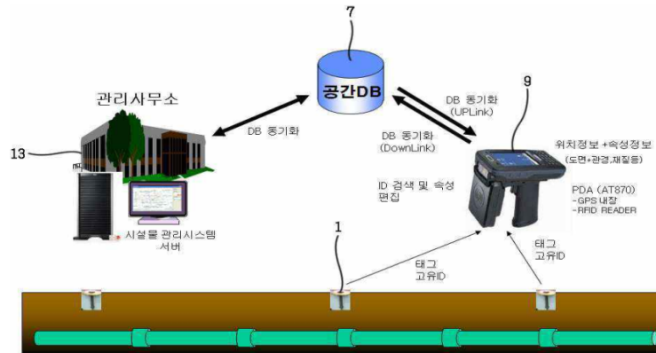
<시설물 관리 시스템의 구성도>
